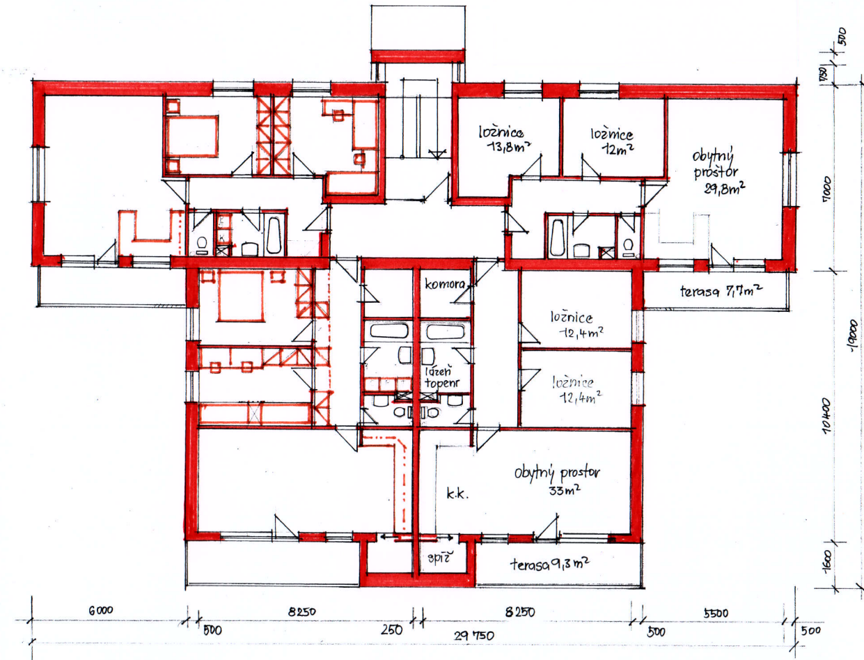
půdorys 1. a 2. N.P.
